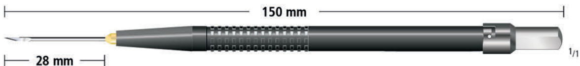
Messer für die Retina-Chirurgie knife for retinal surgery
